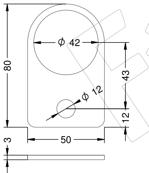
Pletina de anclaje
