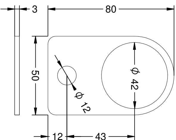
Pletina de anclaje
