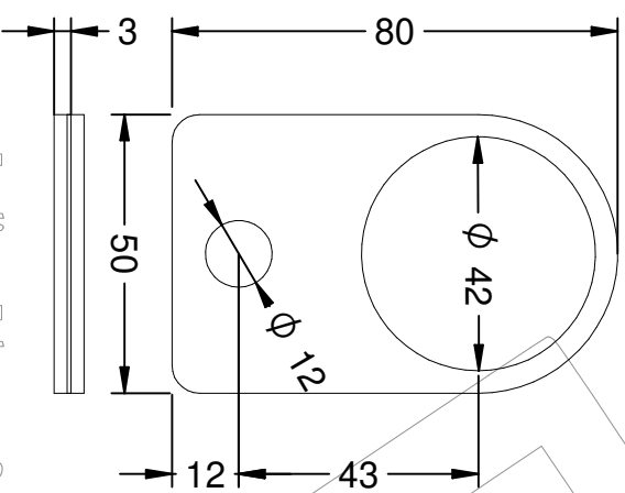
Pletina de anclaje
